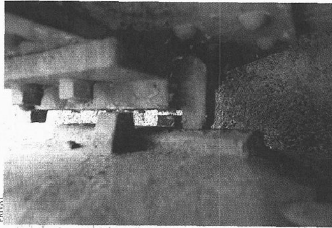
Unbefahrbar: Die Brückenlager wurden aus ihrer Verankerung gerissen
